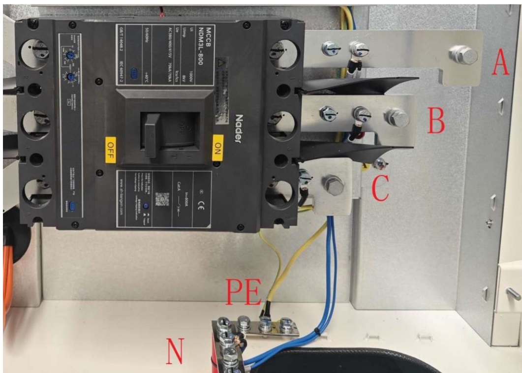
Схема места установки входных кабелей переменного тока зарядной станции
